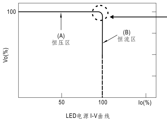
LED电源 I-V 曲线
